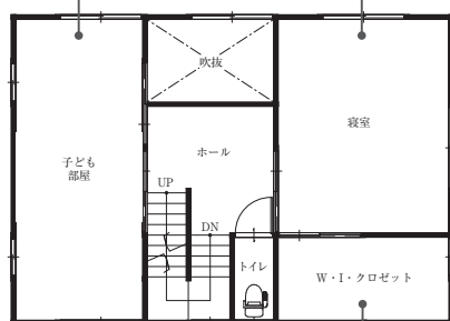
2階平面図
