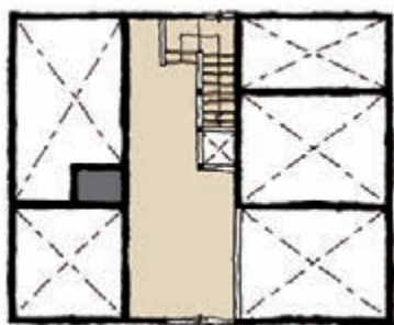
小屋裏平面図
